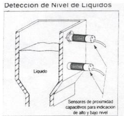
Figura 2. Detección de nivel de líquidos
