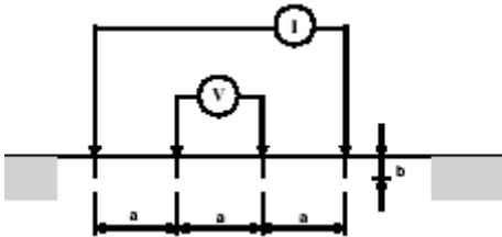
Figura 1. Esquema de medición de resistividad Aparente.
